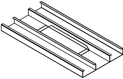
Typ 2 L mit Aufkantung, mit Verstärkung längs
